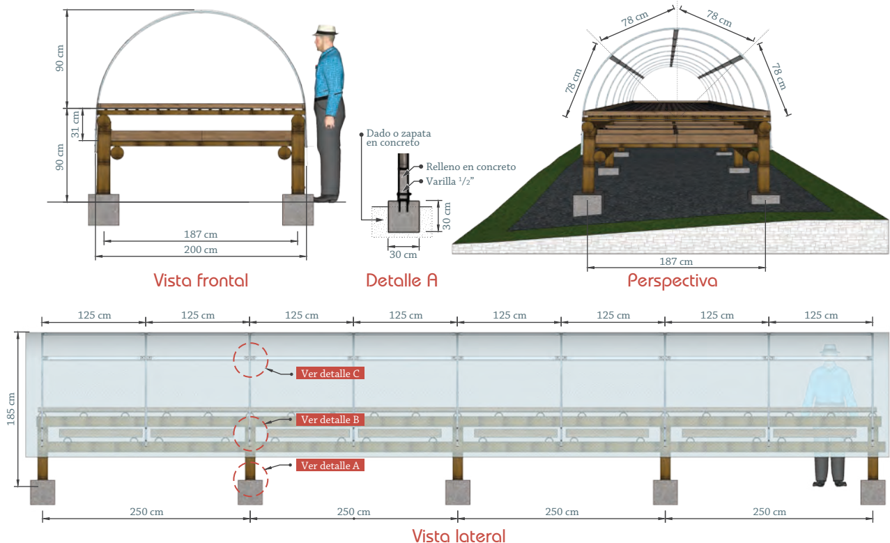
Figura 5. Colocación de los arcos utilizados para la cubierta del secador.
