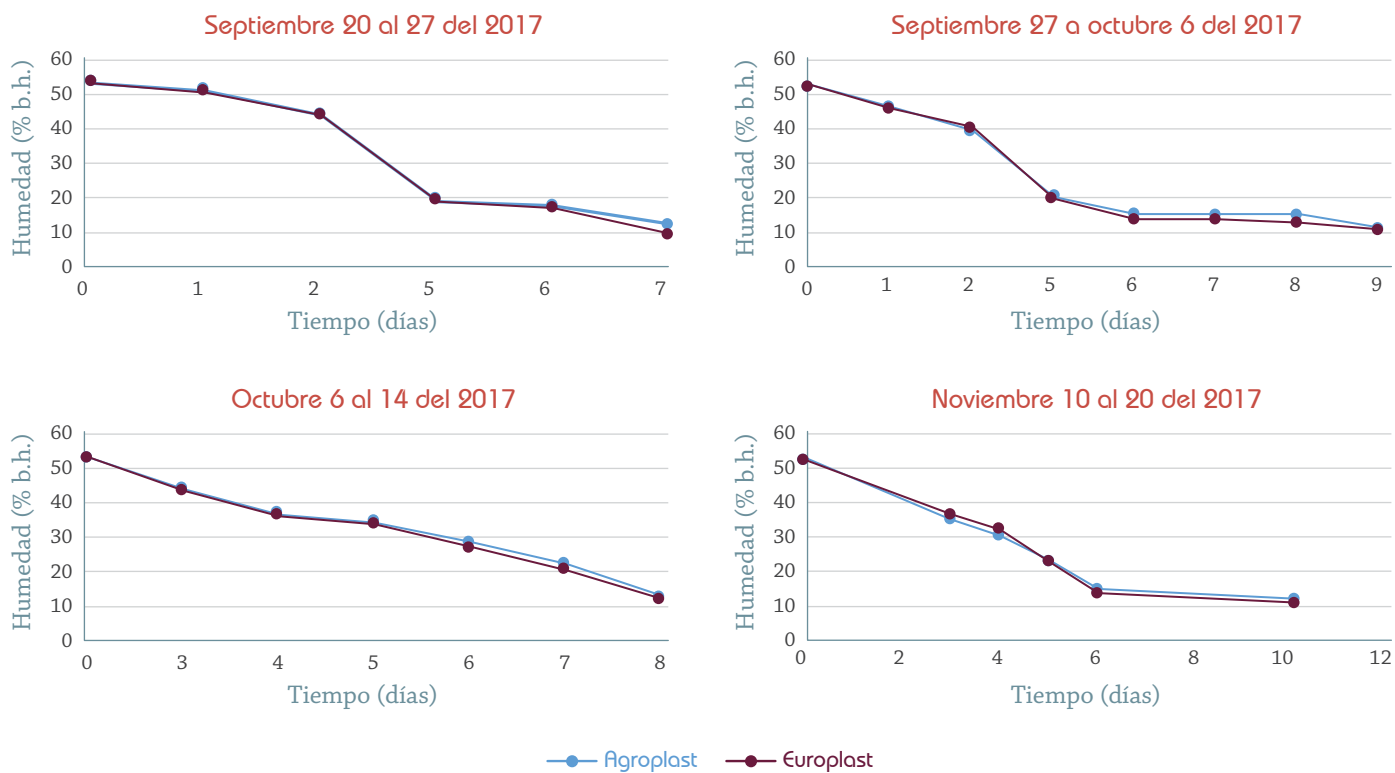
Figura 3. Curvas de secado para café utilizando Agroplast N y Europlast en la cubierta del secador solar tipo túnel obtenidas en Cenicafé (Manizales).
