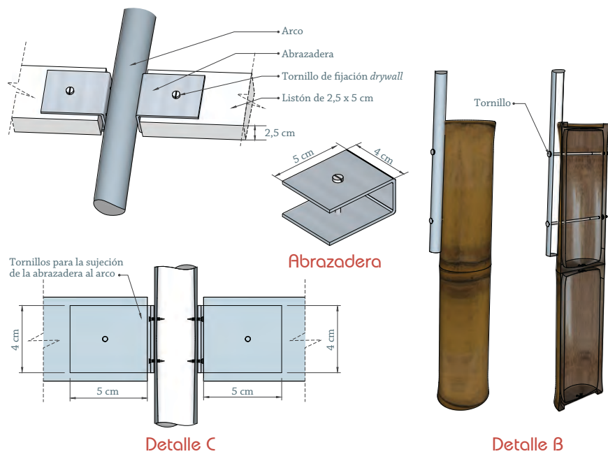
Figura 7. Detalle C, unión de listones a la estructura; Detalle B, unión de arcos metálicos a las columnas de guadua.
