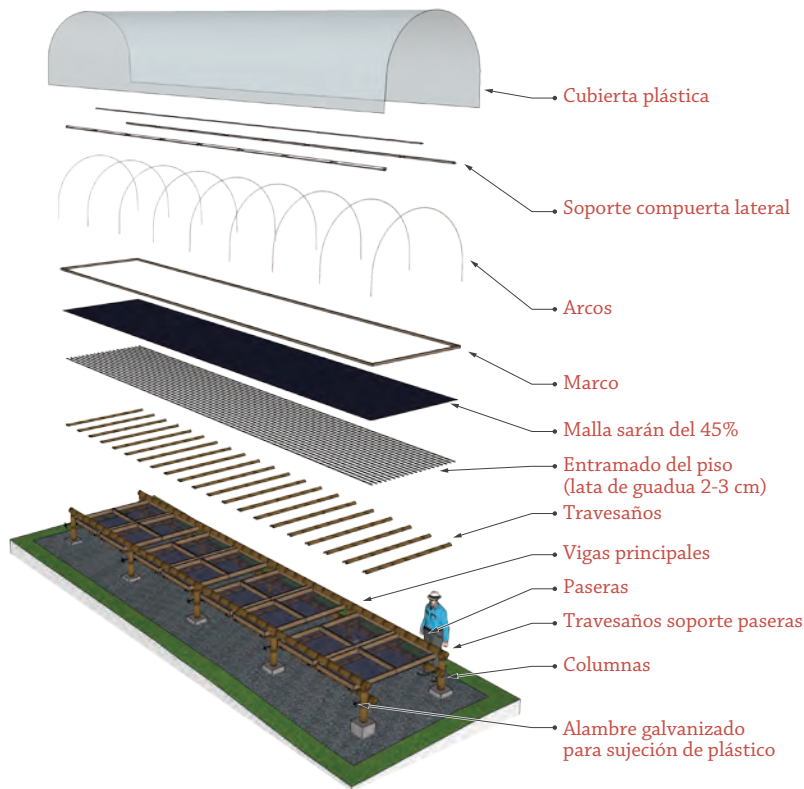
Figura 4. Elementos que componen un secador solar tipo túnel diseñado en Cenicafé. Adaptado de Oliveros et al. (6).
