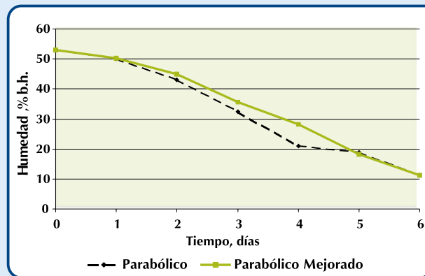
Figura 10. Curvas de secado de café obtenidas con los equipos Parabólico y Parabólico Mejorado
