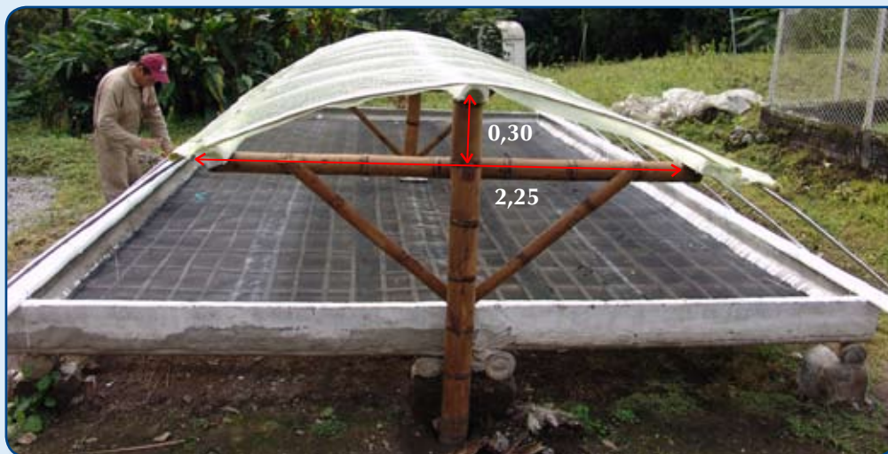
Figura 3. Cumbre o caballete en plástico de la sección parabólica.
